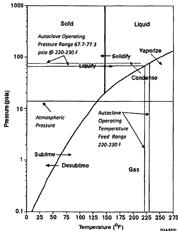
UF_6 Phase Diagram
