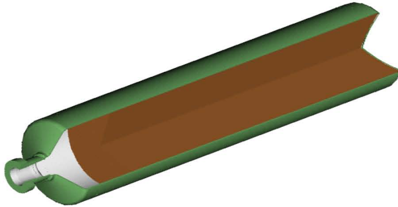
Figure 44. DHLW Glass Pour Canister
