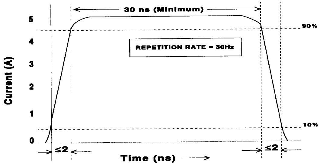
Fig. 6.7. CS115 test signal.
